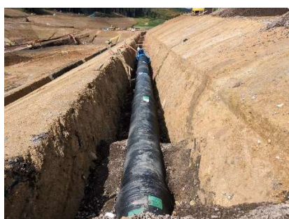
浸出水集排水管 (施工中)
